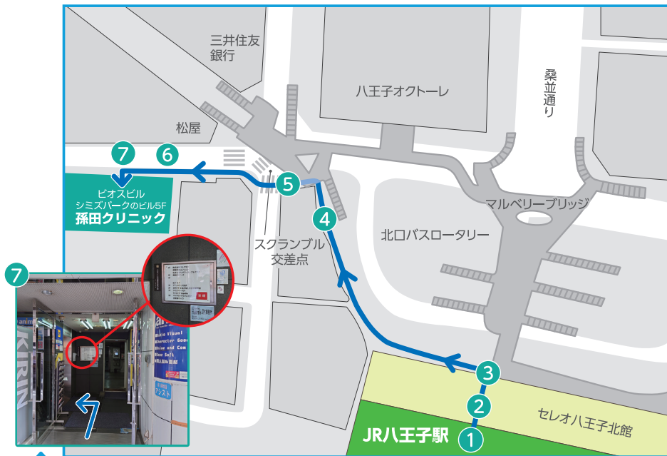
拡大図
