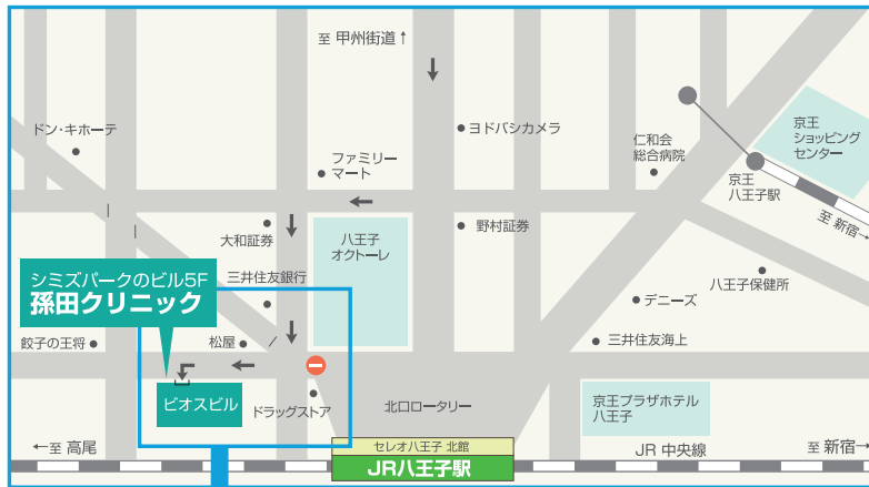
拡大図
